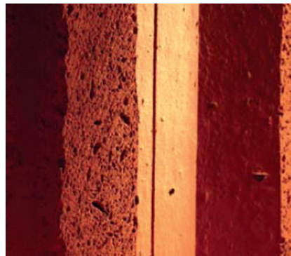
Рис. 6. Поризованная структура черепка
